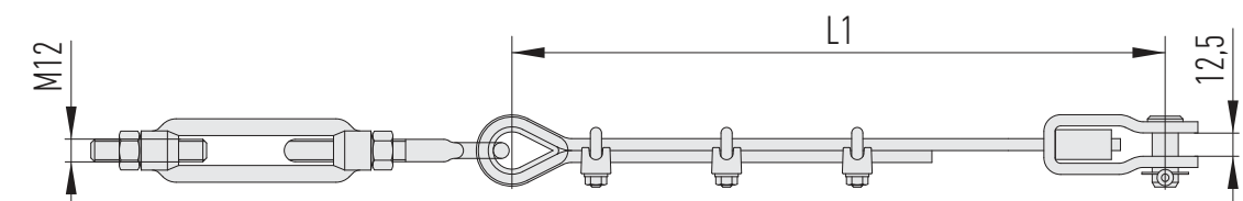
Für 2-Rad-Betätigung/Einachsler
