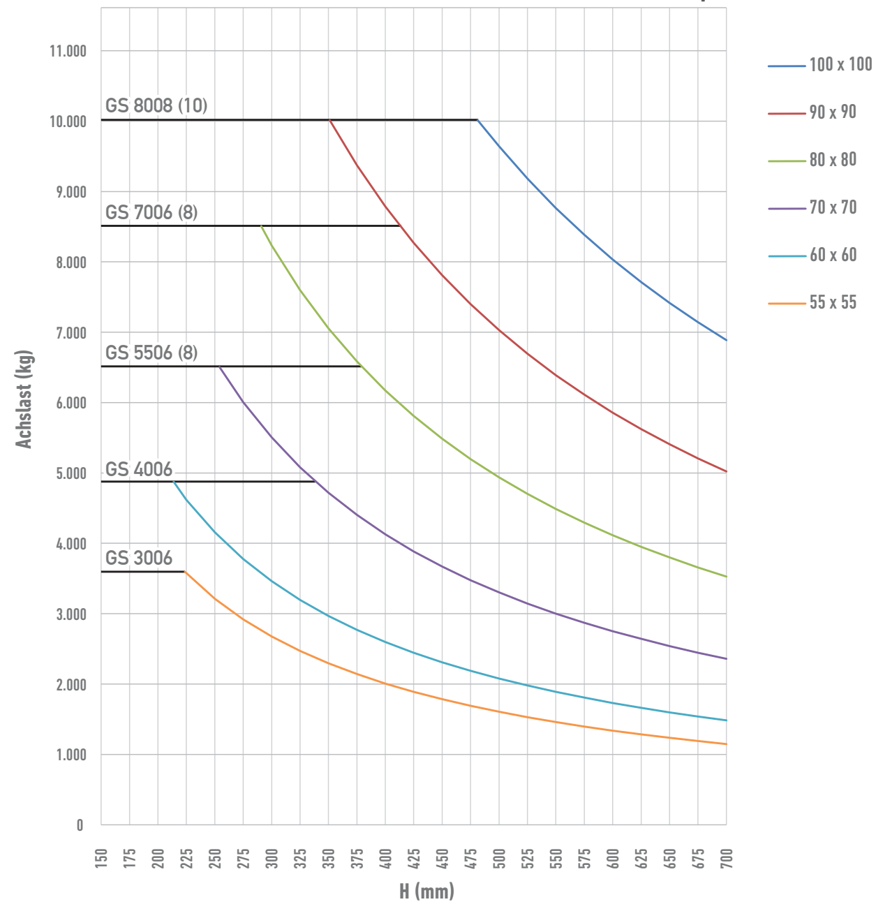
Massivachskörper
