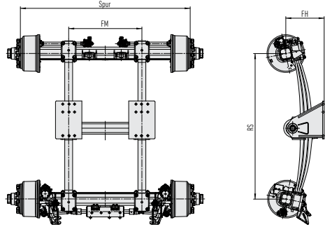
Doppelachsaggregat
