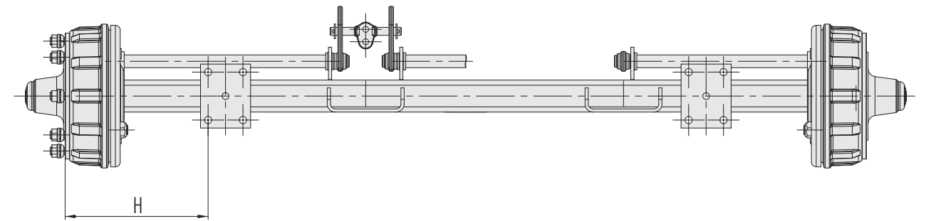
Hohlachskörper
